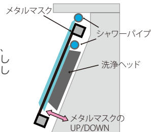
ミスプリント基板セット例 (アダプター使用)
